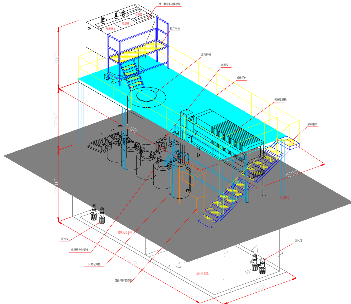
塗裝循環水零排放設備立體圖 (二)
